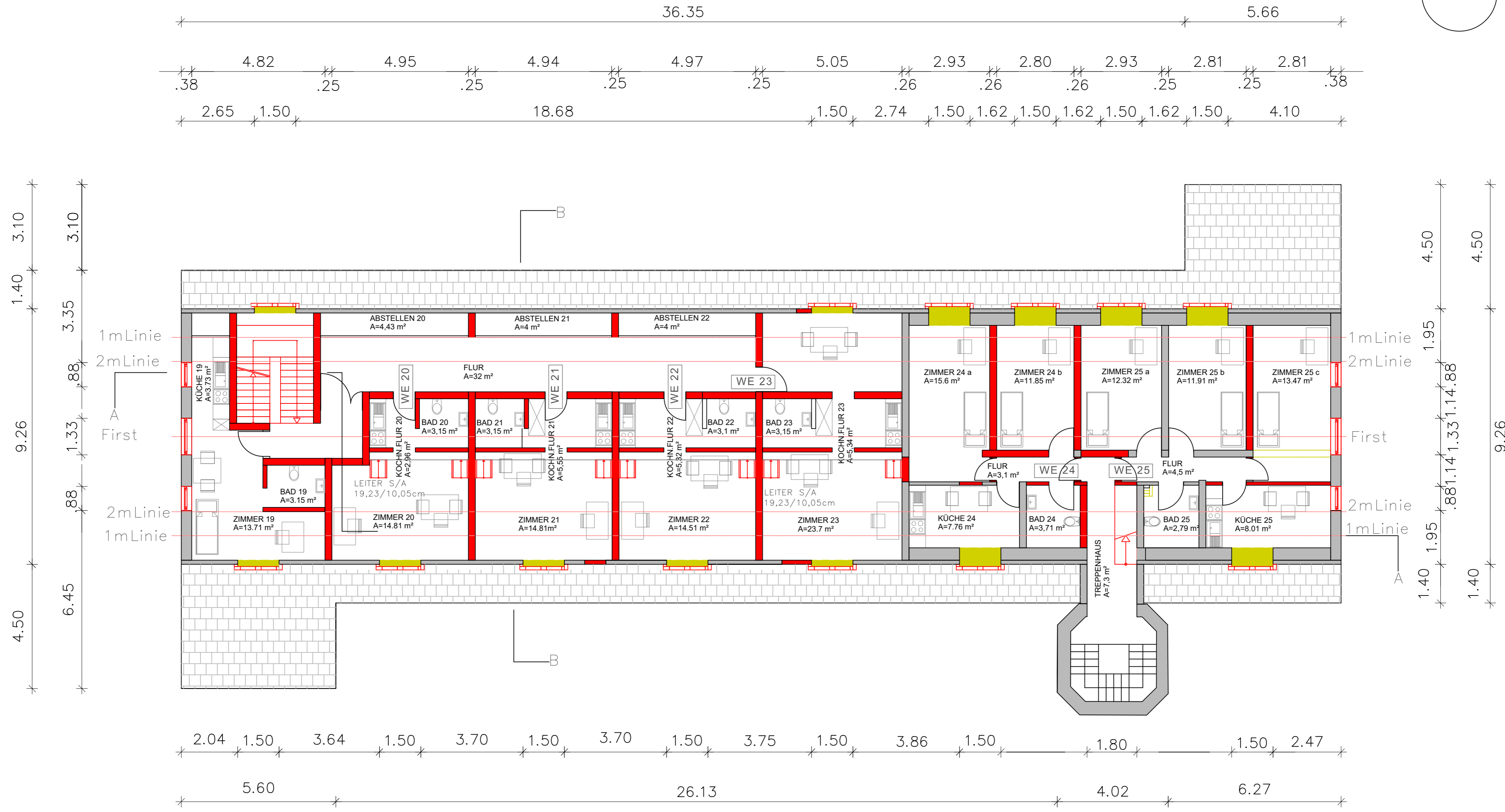
GRUNDRISS DACHGESCHOSS M 1:100 11.07.2018
